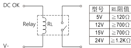
(c) 继电器
